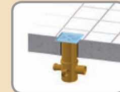
6. Ajuste final a la altura de la cerámica utilizando porta-rejilla macho o acanalado.
