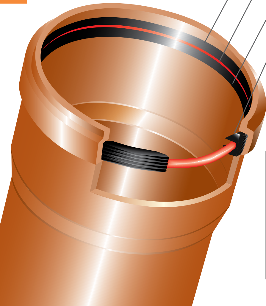
Corte transversal del exclusivo O'Ring de doble labio M.O.L.
