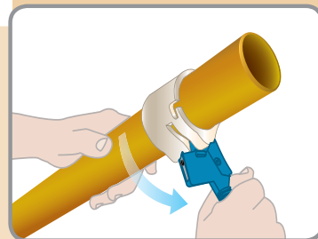
3. Sujete firmemente el tubo y gire la herramienta hasta obtener el corte.
