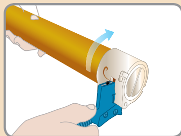
5. Gire la herramienta hasta obtener el refilado.
