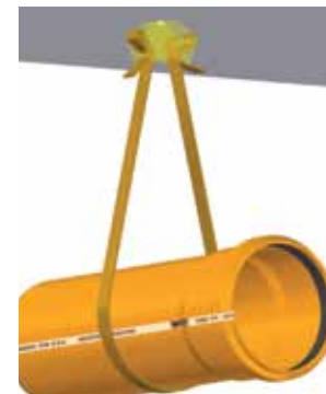
Sujeción doble de tubo Ø 110, fijando la hebilla GrampaFlex en forma directa.
