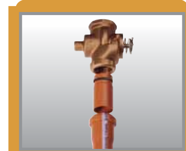
Adaptador 38 x 40 mm acoplado a válvula de inodoro.
