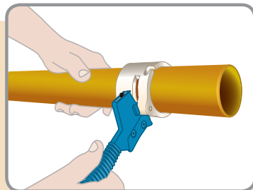
2. Marque la superficie del tubo donde desea realizar el corte. Inserte la herramienta y posicione la cuchilla sobre la marca de corte.
