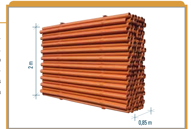
0,85 m de ancho x 2 m de alto = 544 tubos (Ø 110/63/50/40 mm)
